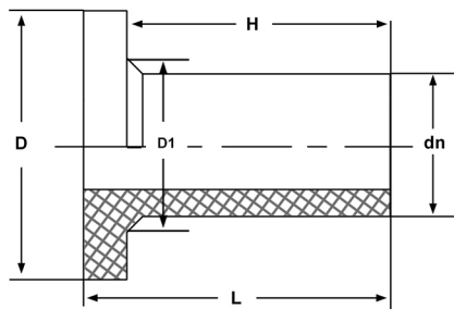
法兰 Stub End
