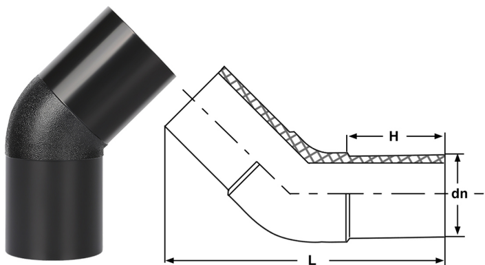
45°弯头 45° Elbow
