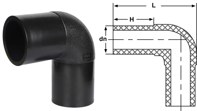
90°等径弯头 90° Elbow
