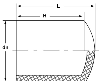
管帽 End Cup
