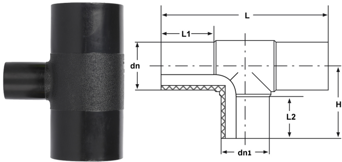
异径三通 Reducing Tee
