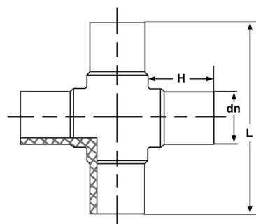
四通 Cross Tee
