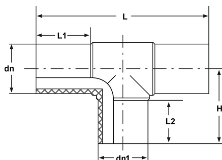
异径三通 Reducing Tee
