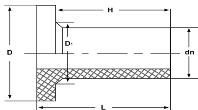
长颈法兰 Stub End Long Neck
