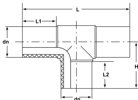
等径三通 Equal Tee
