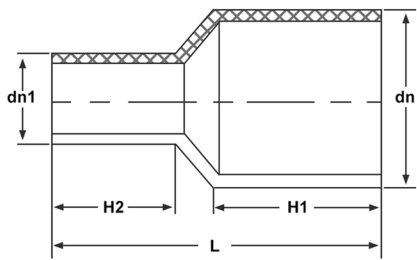
异径直接 Reducer
